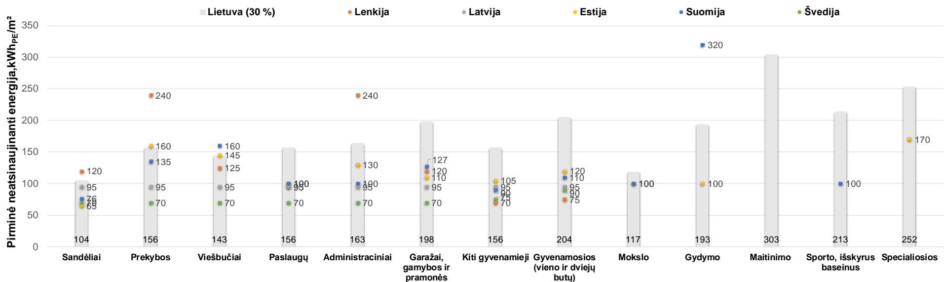
3.4 pav. 30 % efektyviausiems pastatams Lietuvoje ir kitose šalyse naujiems pastatams nustatytų pirminės neatsinaujinančios energijos reikšmių palyginimas
